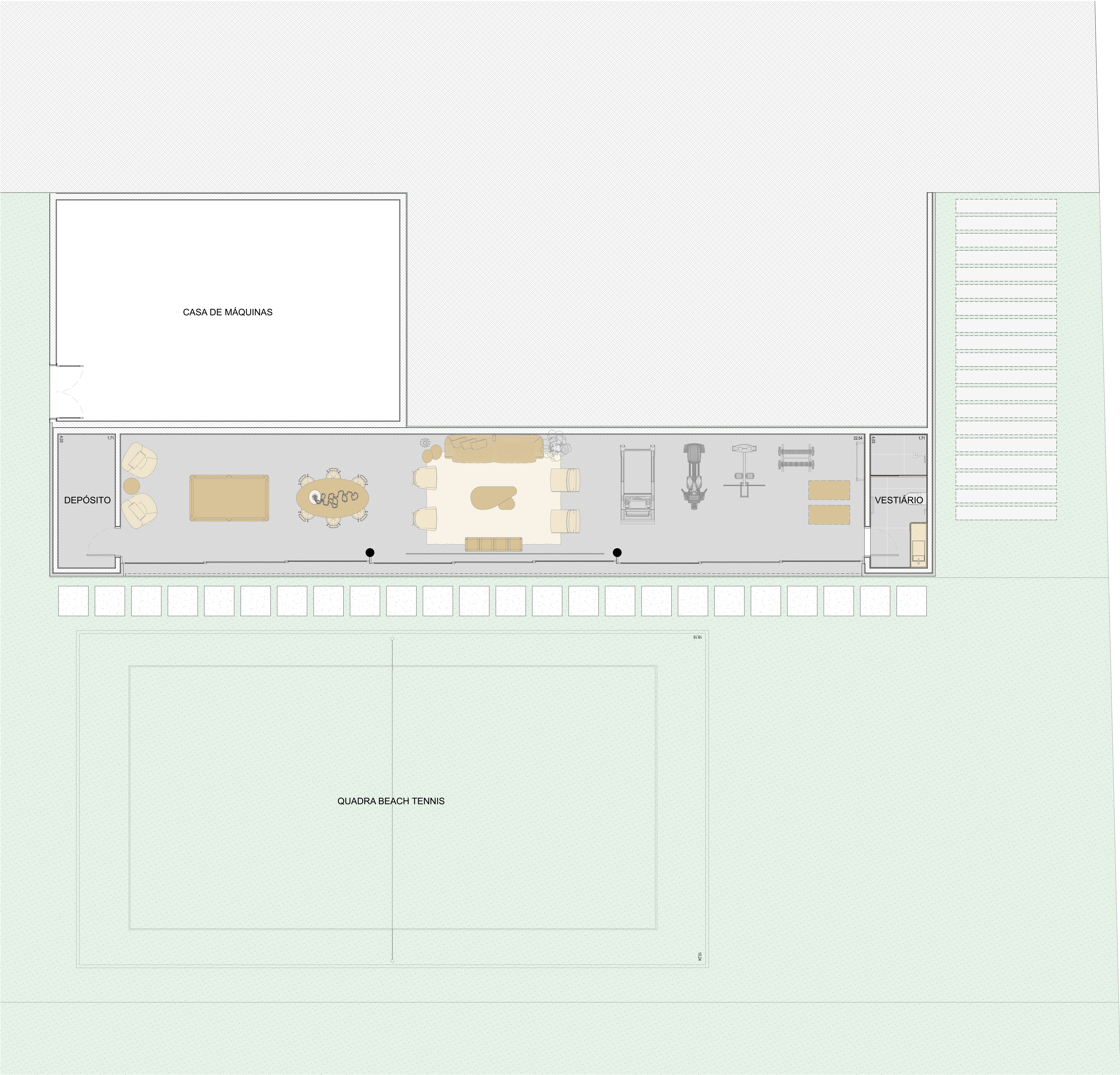
PISO INFERIOR Esc: 1:50
